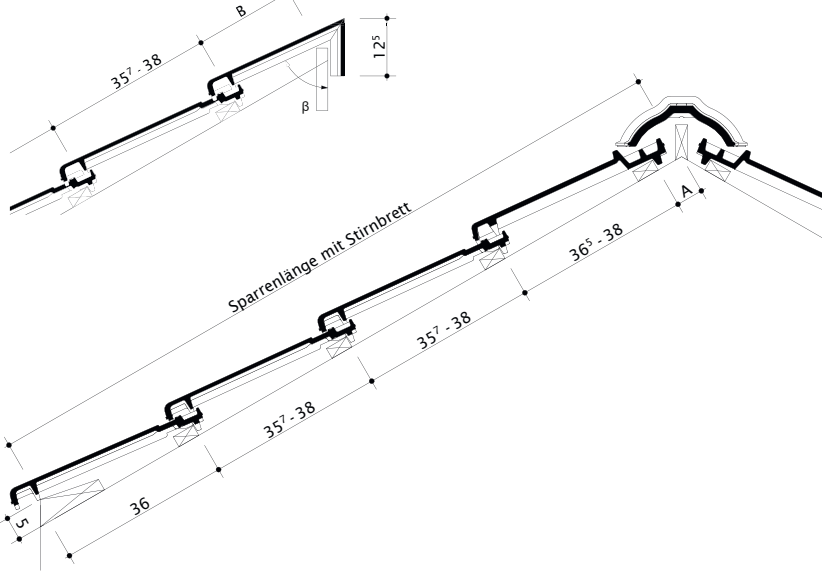
Längsschnitt MST 1/15
