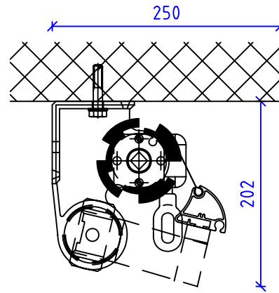
DECKENMONTAGE
