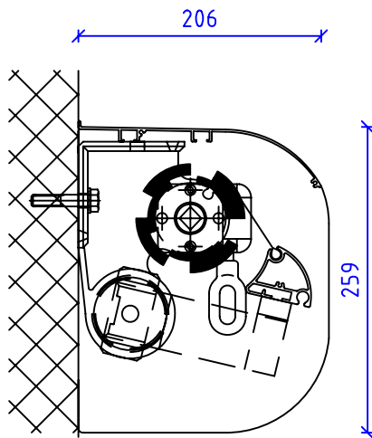
WANDMONTAGE MIT SCHUTZDACH
