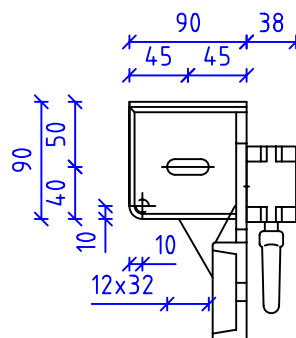
KONSOLE ANSICHT VORNE
