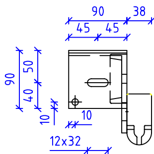
KONSOLE ANSICHT OBEN
