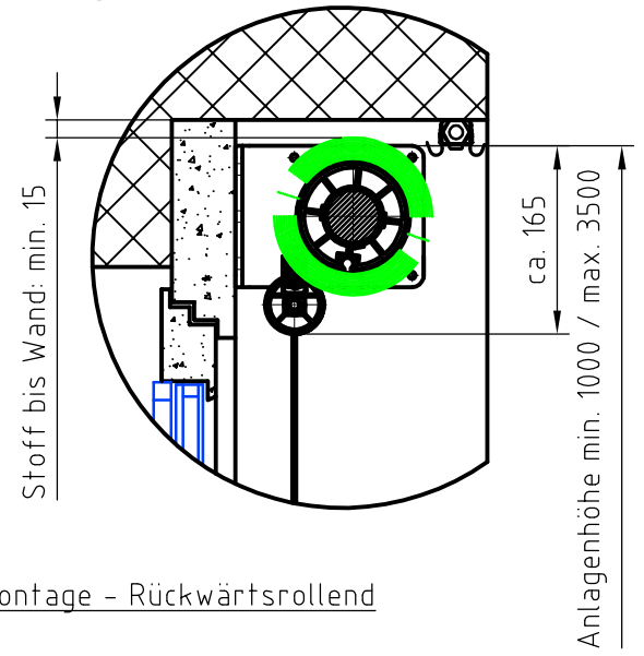
Fassadenmontage
