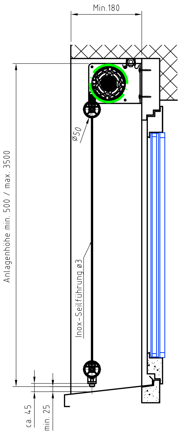
Fassadenmontage - Vorwärtsrollend
