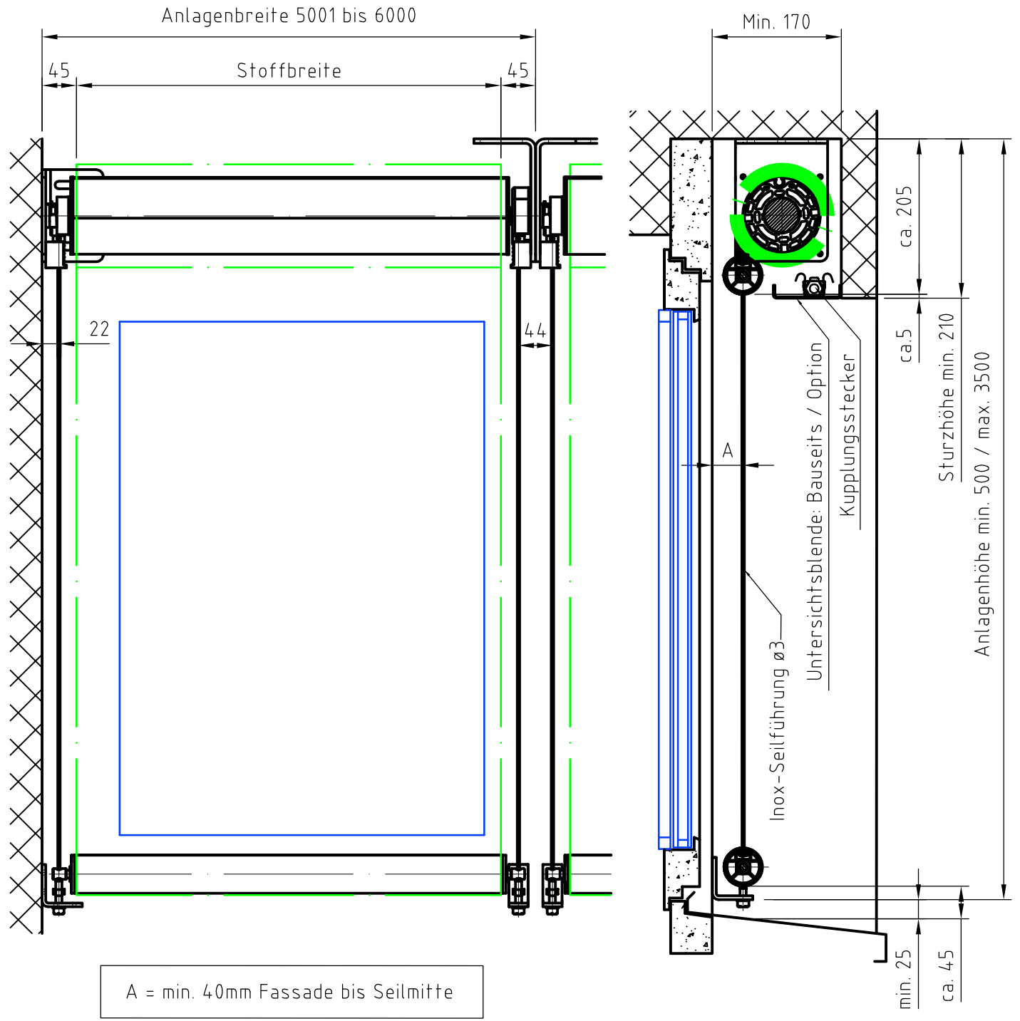
Deckenmontage - Rückwärtsrollend
