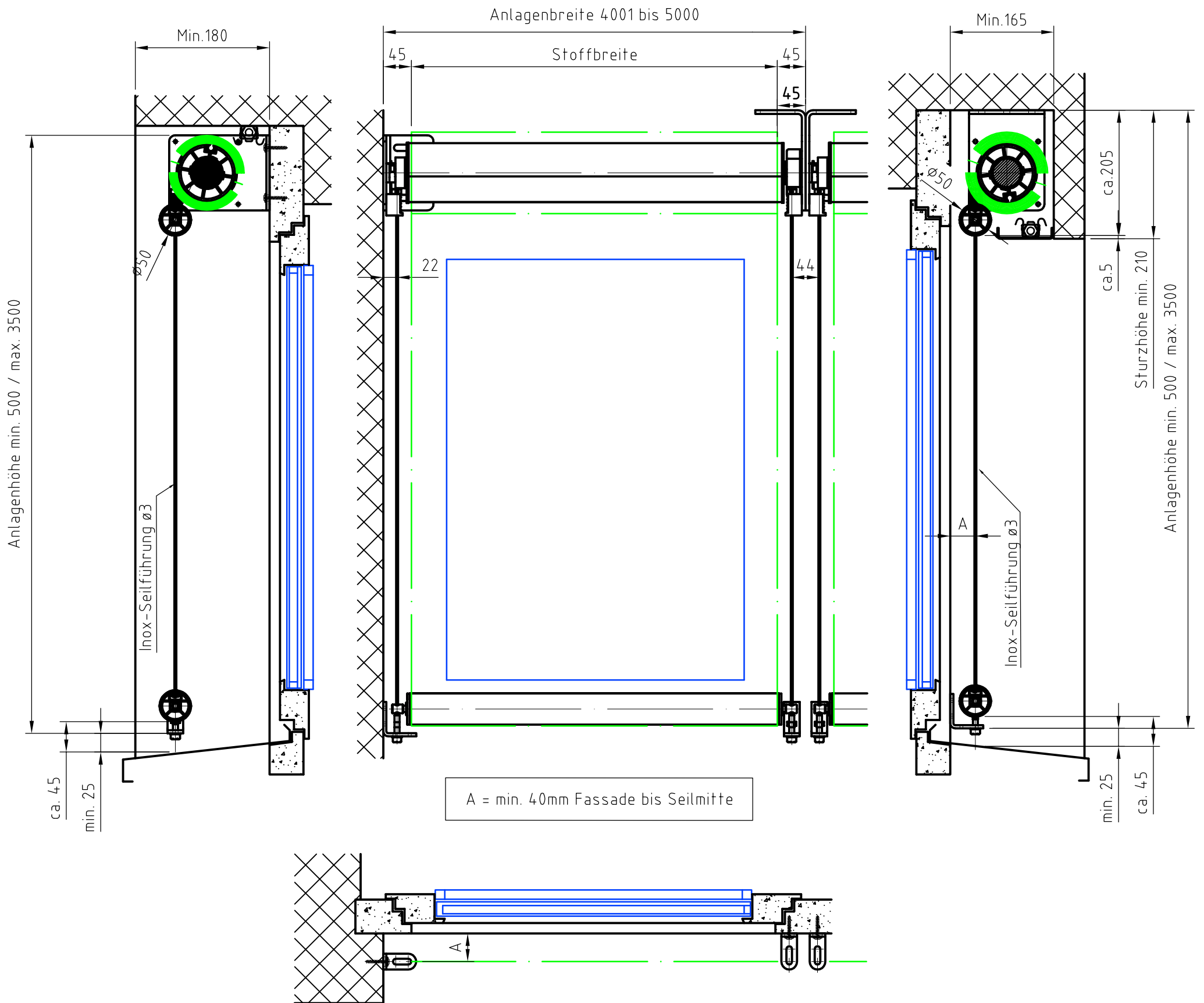
Fassadenmontage - Vorwärtsrollend
