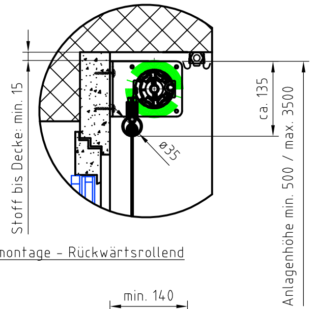
Fassadenmontage
