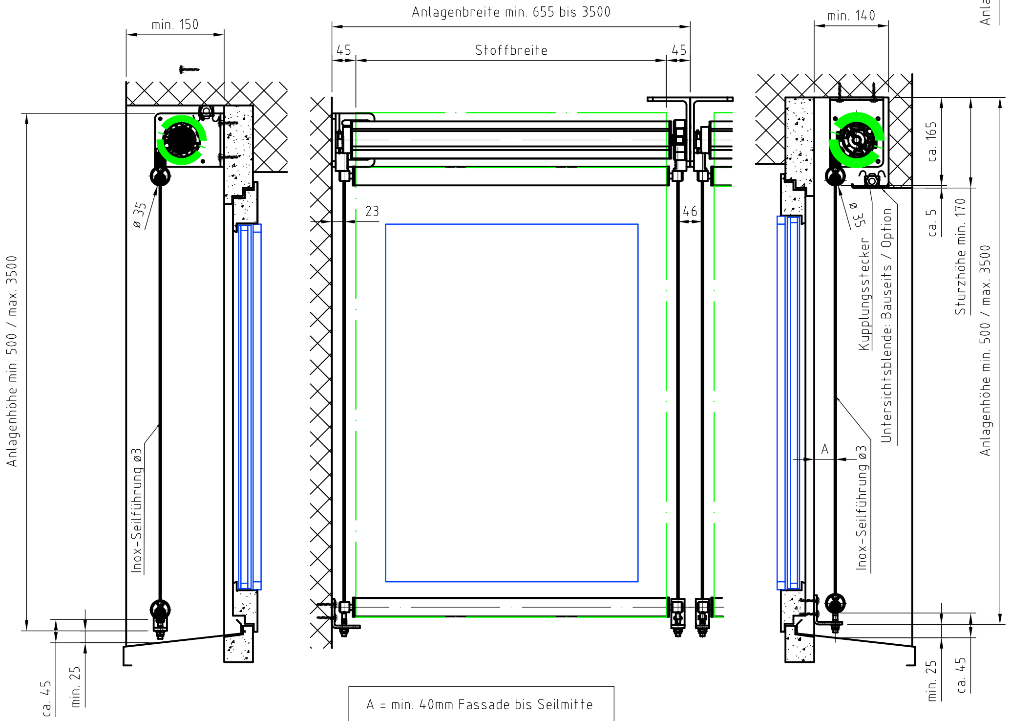
Fassadenmontage - Vorwärtsrollend
