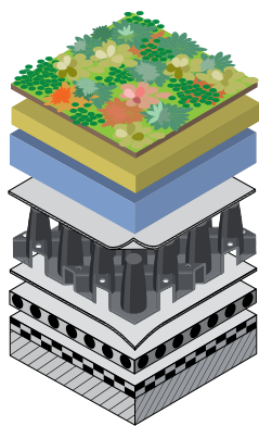
Aufbau Nophadrain Extensiv Grunddachsystem mit ND 6+1v
