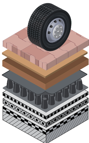
Aufbau Parkdachdachsystem - Lkw (Belastungsklasse 3) mit ND 620hd
