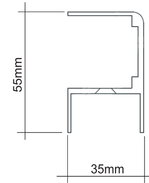
Ecke 90°
