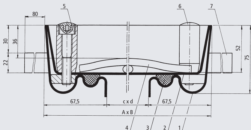
Tipo BVE Edelstahl, Scala 1 : 2,5
